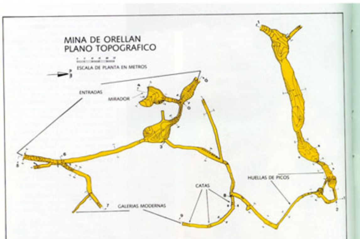
PLANTA DE LA MINA JUNTO AL MIRADOR DE ORELLAN (Bibl. David Gustavo López. Dib. Toño)
